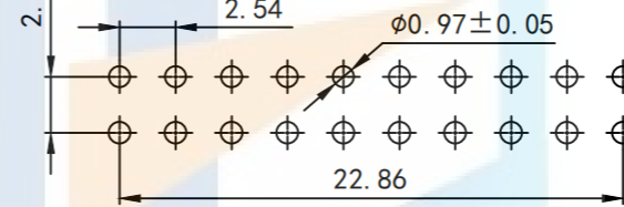
PCB开孔
