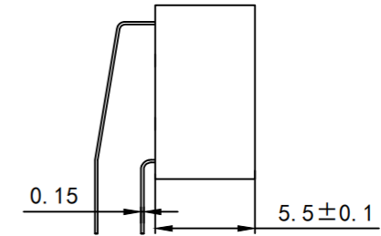
平推钮 (R)
