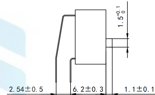
高推钮 (E)
